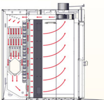
Vitesse lente de 8 à 12 mètres par seconde en fonction des modèles de four. → Flux d'air chaud
