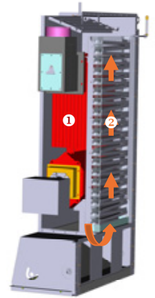
Appareil à buée constitué de gouttières en fonte
